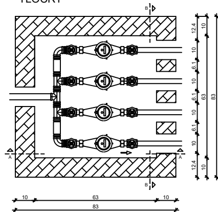
TLOCRT
