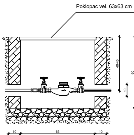
PRESJEK A-A
