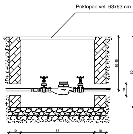
PRESJEK A-A
